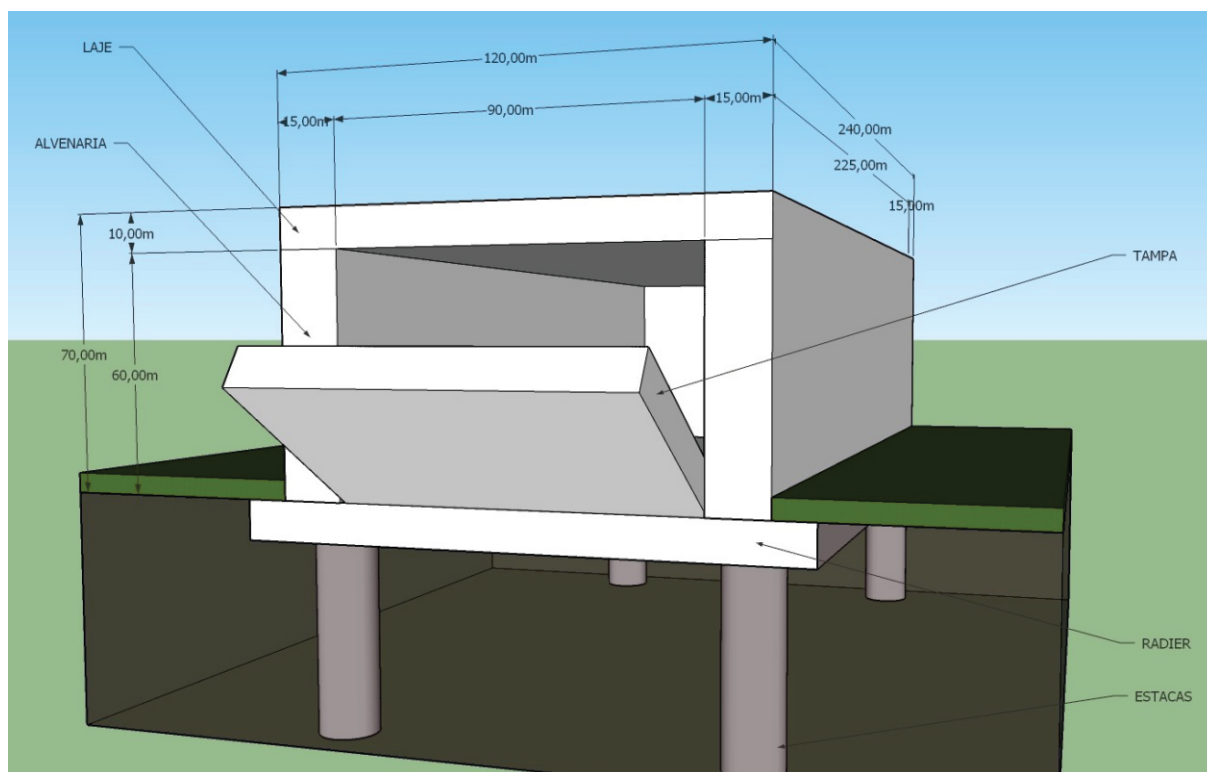
TERRENO 1,20x2,40m | MODELO 1
