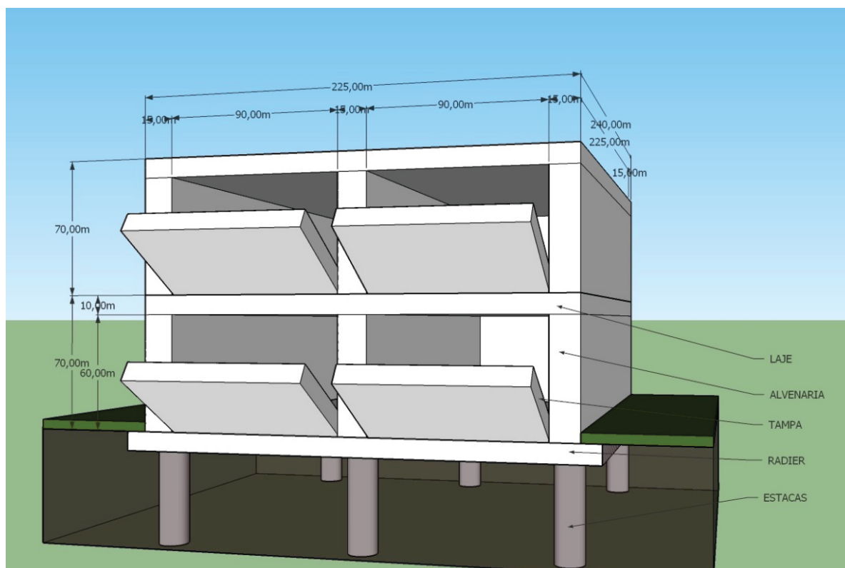
TERRENO 2,40x2,40m | MODELO 2
