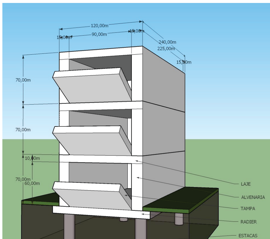
TERRENO 1,20x2,40m | MODELO 3
