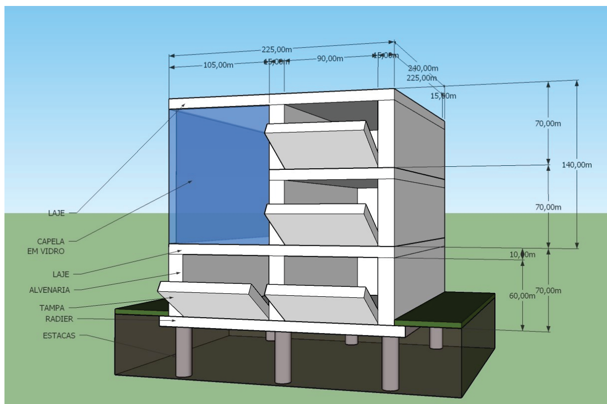
TERRENO 2,40x2,40m | VARIAÇÃO 2
