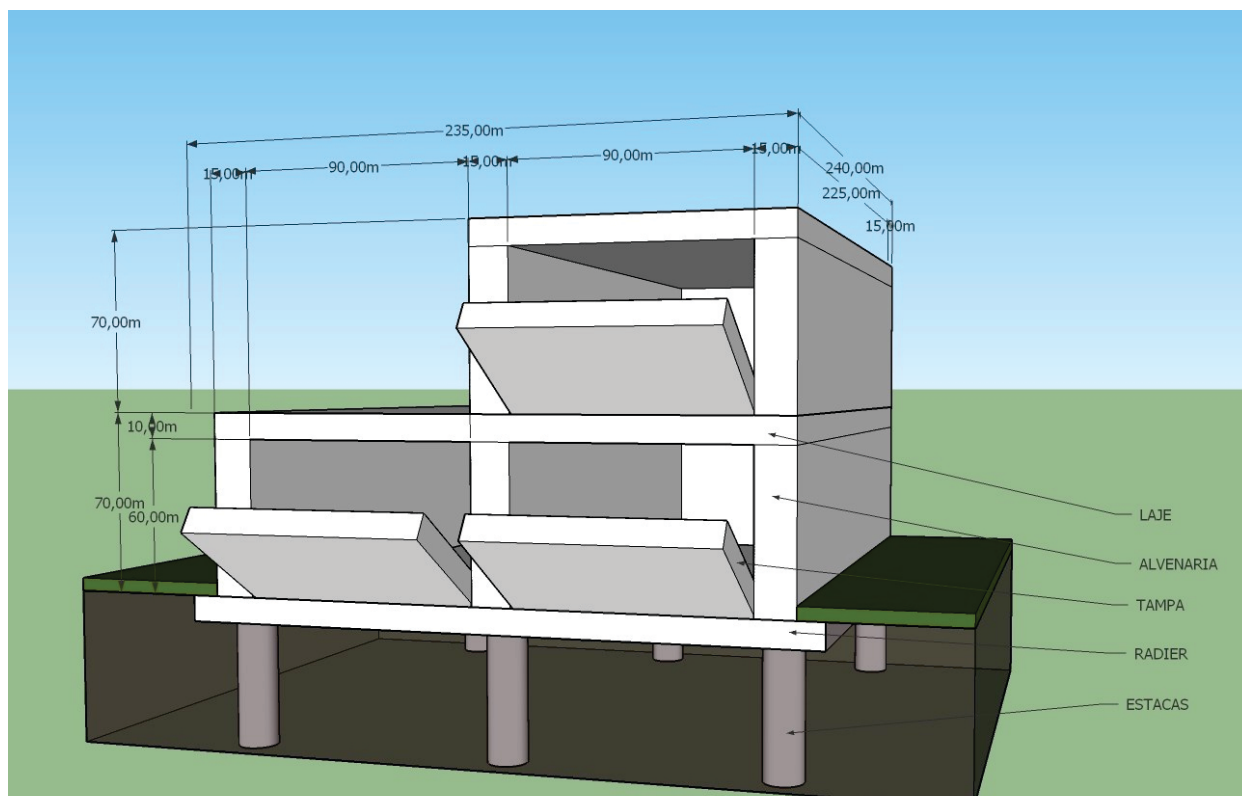
TERRENO 2,40x2,40m | VARIAÇÃO 1
