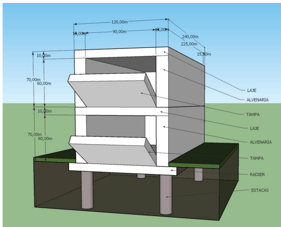
TERRENO 1,20x2,40m | MODELO 2
