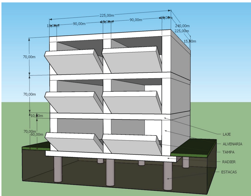
TERRENO 2,40x2,40m | MODELO 3
